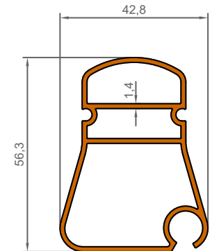
1001 0,916 KG/M
