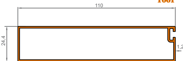
1133 0,897 KG/M
