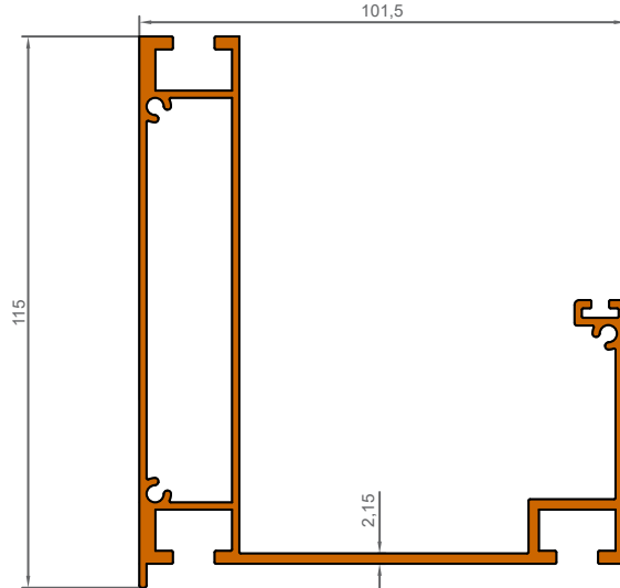
1013 2,307 KG/M
