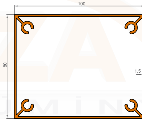
1121 1,986 KG/M
