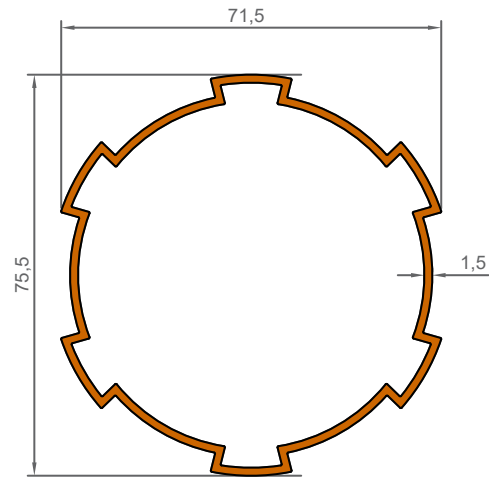
1007 1,076 KG/M
