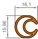
1009 0,231 KG/M
