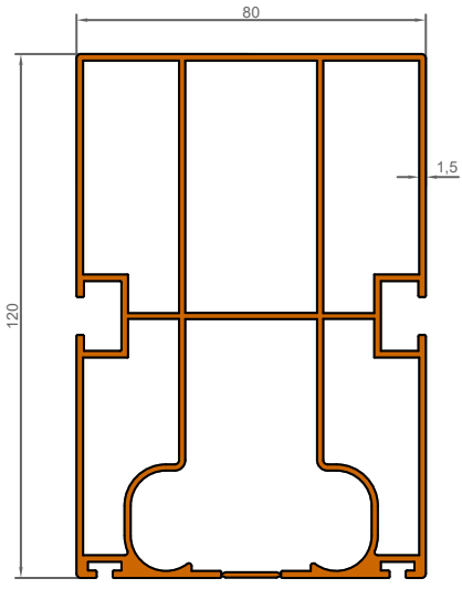
1011 3,141 KG/M
