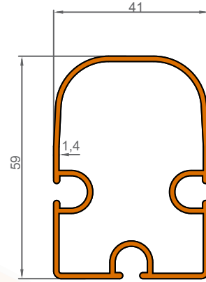
1137 0,886 KG/M
