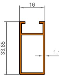
1010 0,307 KG/M
