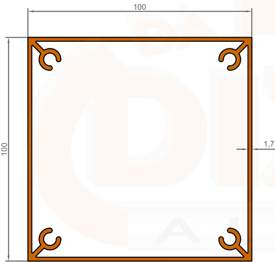
1012 2,377 KG/M
