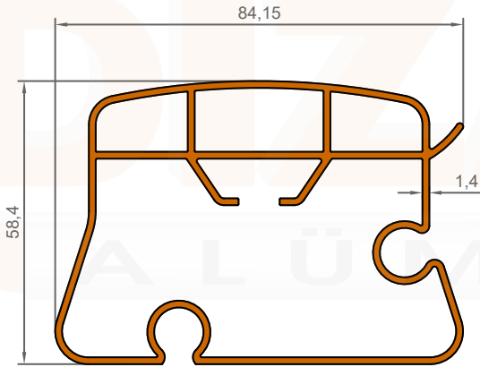
1004 1,635 KG/M
