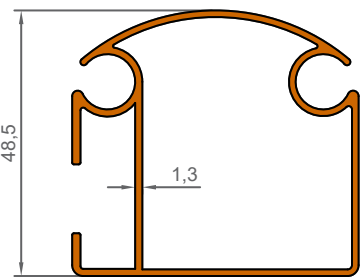
1008 0,813 KG/M
