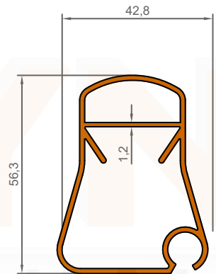
1002 0,865 KG/M
