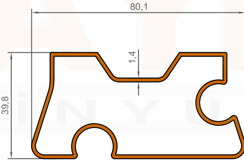
1005 1,011 KG/M
