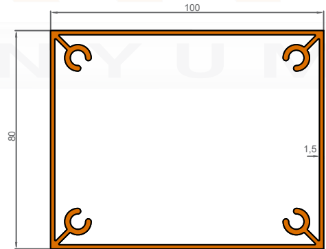
1121 1,986 KG/M
