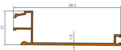
1015 0,748 KG/M
