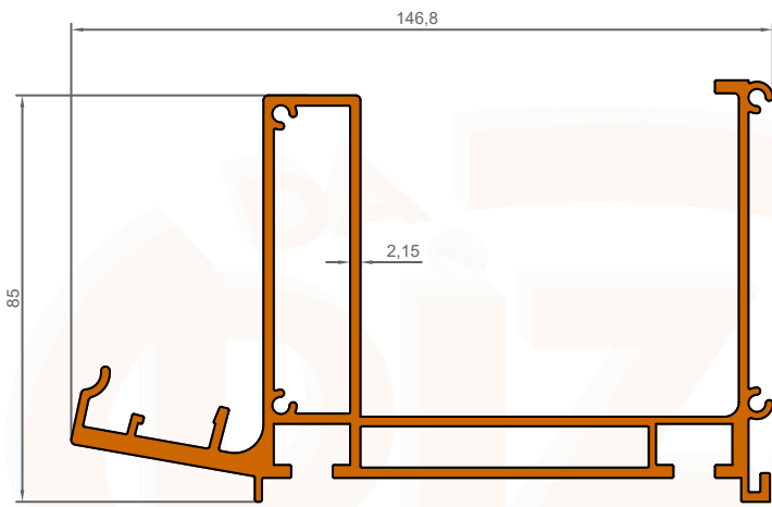
1033 3,380 KG/M
