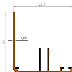
4007 0,632 KG/M
