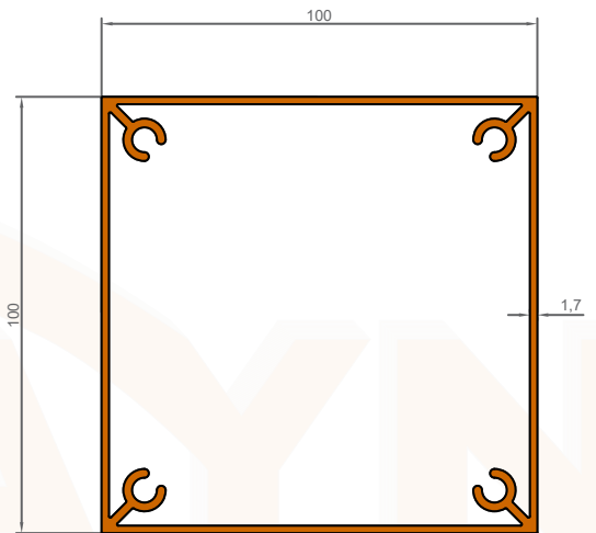
1012 2,377 KG/M
